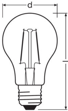
P RF CLAS P 7 W/827 E27
