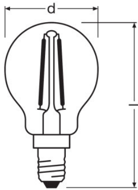
P RF CLAS P 1.6 W/827 E14
