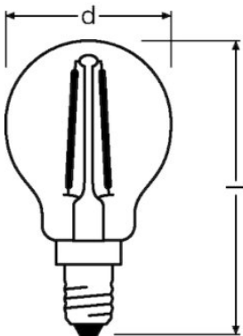
P RF CLAS P 2.5 W/827 E14
