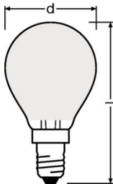
P RF CLAS P 4 W/827 E14, P RF CLAS P 40 4 W/827 E14
