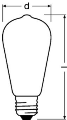
P RF CLAS GL 4.5 W/827 E27, P RF CLAS GL 7 W/827 E27
