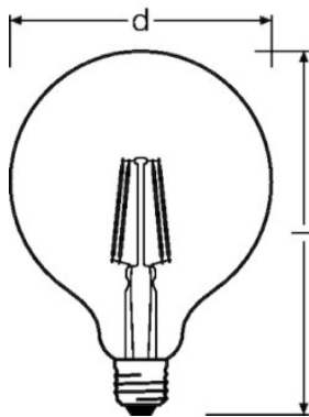
P RF CLAS GL 4 W/827 E27, P RF CLAS GL 6.5 W/827 E27
