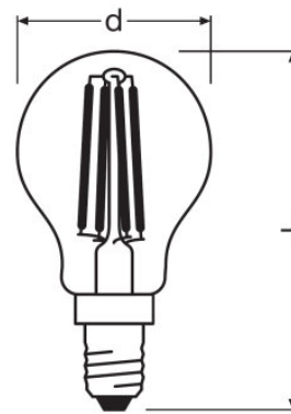
SST CLAS A 4 W/827 E14
