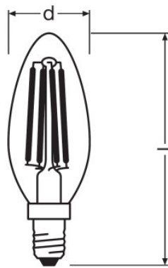
SST CLAS A 4 W/827 E14
